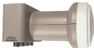
LNB QUAD VHVH Out: 4 VHVH Guadagno: 60dB cod. 80188KL
