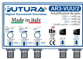
AMPLIFICATORE VHF-UHF 2x UHF 5-30 dB - BIII 5-20 dB 2 OUT = 110dBμV cod. AR3VUU2
