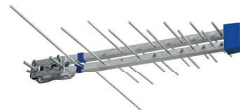
ANTENNA LOG 16 elementi Guadagno: 13dB cod. LP16/345MINI
