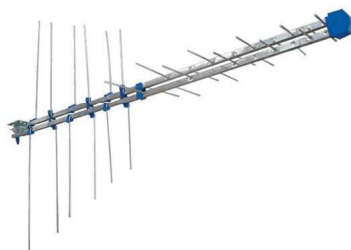
ANTENNA LOG 16 elementi Guadagno: 9,5dB cod. LP16/HV
