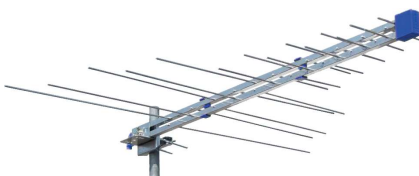
ANTENNA LOG 16 elementi Guadagno: 13dB cod. LP16/345
