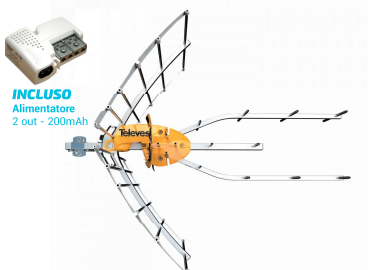
ANTENNA BOSS UHF 470 - 790 MHz Guadagno: 38±2 dB cod. 148902
