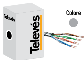
Cavo Dati U/UTP - Bobina 305mt Cat-5E - Eca LSFH cod. 219602
