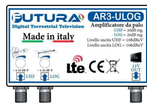
AMPLIFICATORE LOG 2 IN reg. | LOG 20dB - UHF 20dB 1 OUT 108 dBμV cod. AR3ULOG
