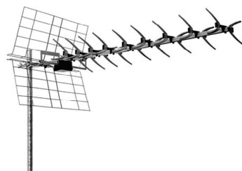
ANTENNA UHF 41 Elementi Guadagno: 14,5dB cod. 40XWL
