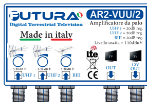
AMPLIFICATORE VHF-UHF 2x UHF - BIII (5-20 dB) 2 OUT = 110dBμV cod. AR2VUU2
