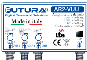
AMPLIFICATORE VHF-UHF 2x UHF - BIII (5-20 dB) 1 OUT = 110dBμV cod. AR2VUU
