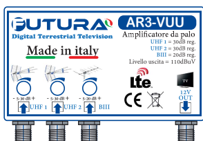
AMPLIFICATORE VHF-UHF 2x UHF 5-30 dB - BIII 5-20 dB 1 OUT = 110dBμV cod. AR3VUU
