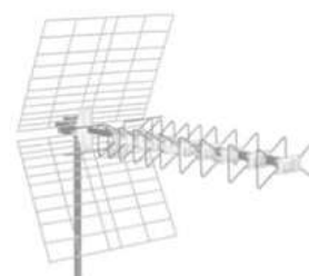
ANTENNA UHF 42 elementi Guadagno: 14dB cod. ANT420FLTE
