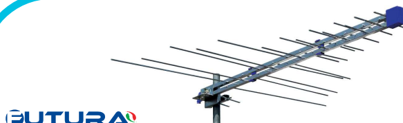
ANTENNA LOG 30 elementi Guadagno: 11dB cod. 560UD
