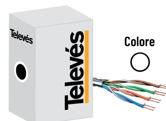
Matassa cavo LAN UTP 5E N. di coppie: 4 Diametro esterno tot.: 5 mm mt confezione: 305 mt cod. LAN1051UTP
