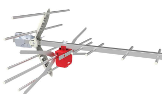
ANTENNA COMBO 5 Elementi Guadagno: 10dB cod. FLYCOMBO
