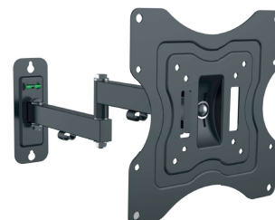
Supporto TV 23" a 42" VESA 200x200 Max 15kg - 3 Snodi cod. 41860
