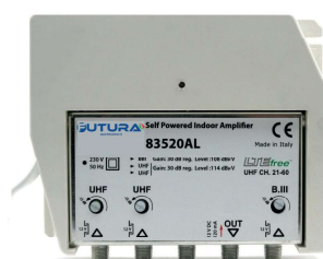
Centralino Autoalimentato 3IN + BIII(30dB reg.) + UHF (30dB reg.) + UHF(30dB reg.) - LIV. USC. 108/114dBuV cod. 83520AL
